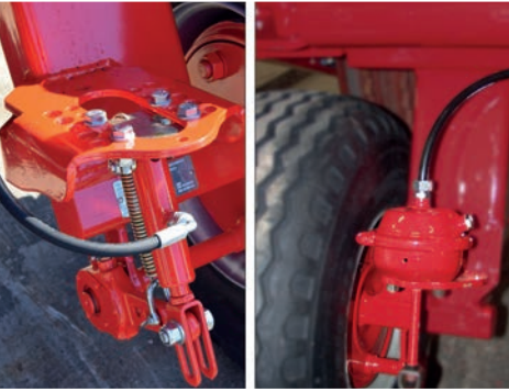
Hydr. / Druckluftbremsanlage
