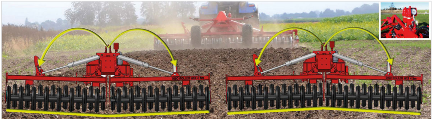
Grundausstattung an 2- und 3-teiligen Modellen: HE-VA SAT-System: Hydr. einstellbares Gewichtsausgleichsystem, gewährleistet einen gleichmäßigen Druck auf der ganzen Arbeitsbreite und so eine optimale Boden Anpassung.
