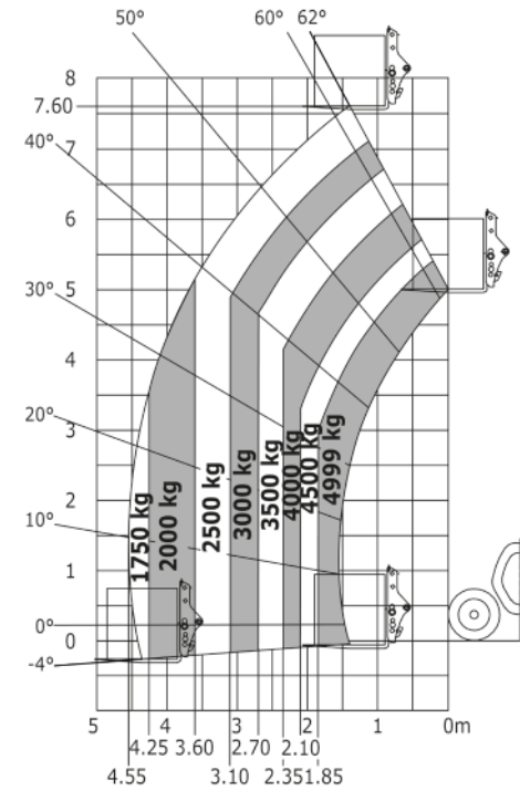
Lastdiagramm Rough-Terrain (EN1459 B) 500 mm Lastschwerpunkt
